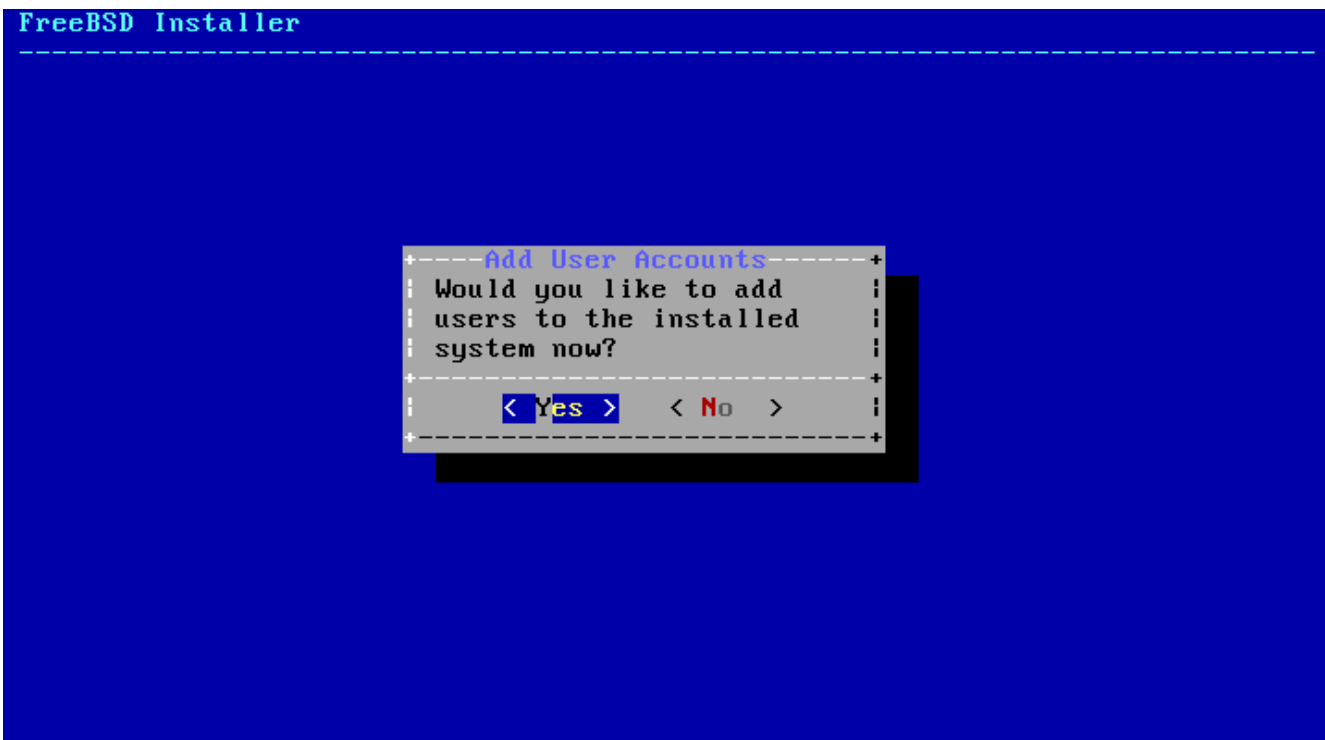
Abbildung 42. Benutzerkonten hinzufügen
