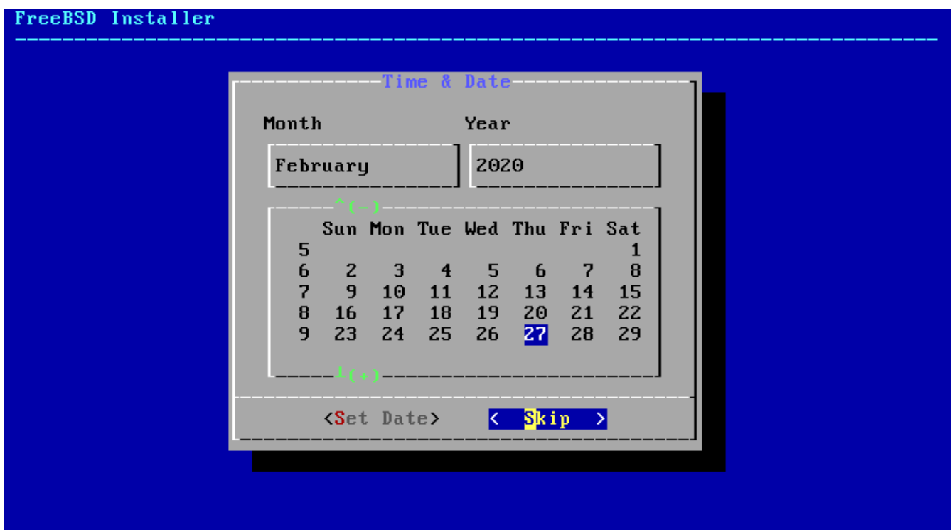
Abbildung 38. Datum auswählen
