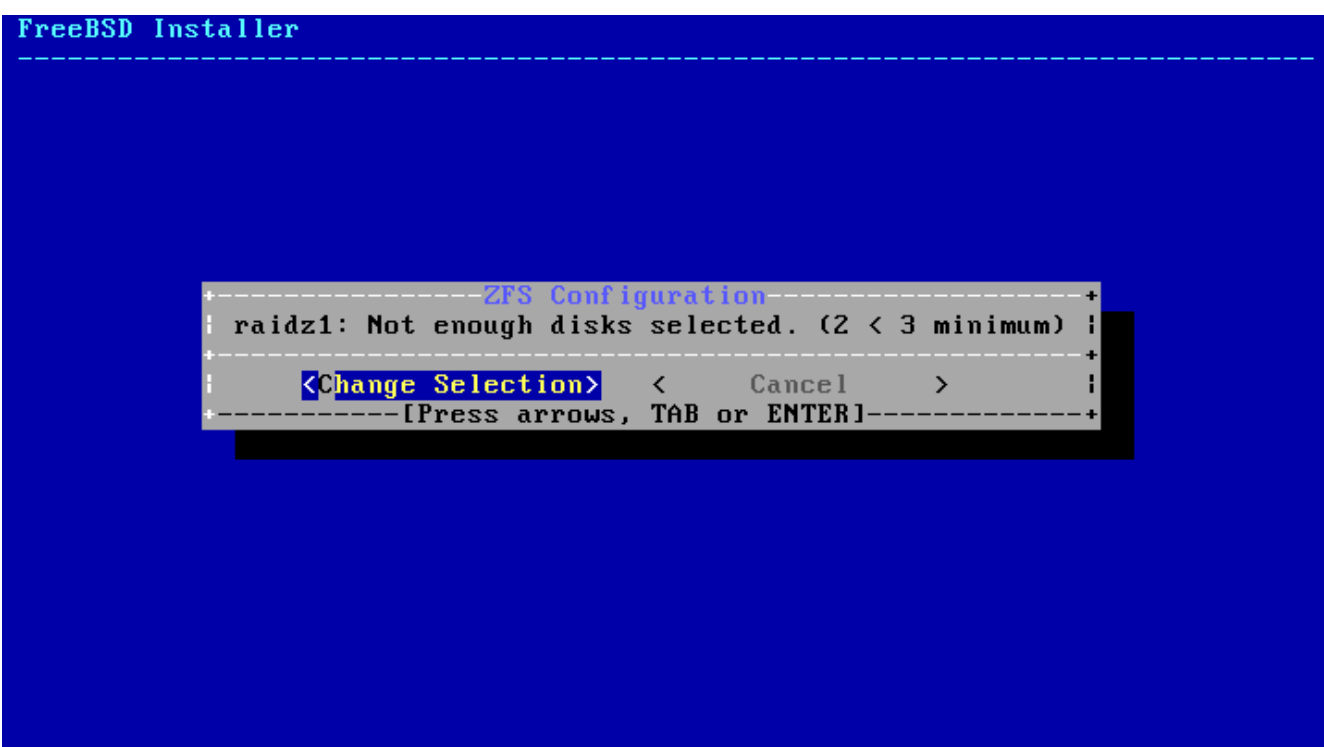
Abbildung 22. Ungültige Auswahl
